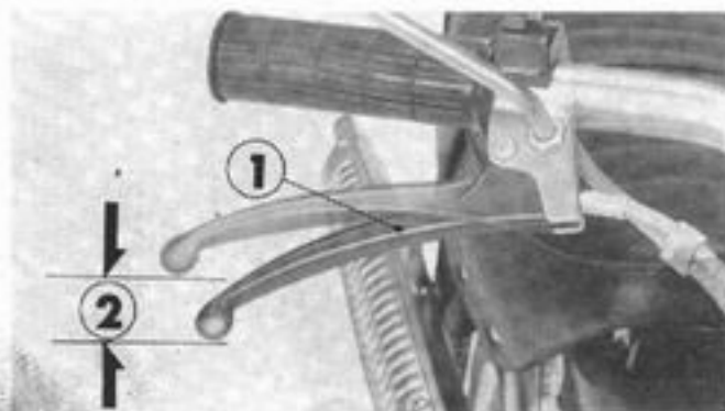
① Poignée de frein avant ② Jeu
