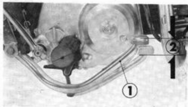
① Pédale de frein arrière ② Jeu
