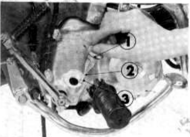
① Bouchon de remplissage d'huile ② Repère supérieur ③ Repère inférieur
